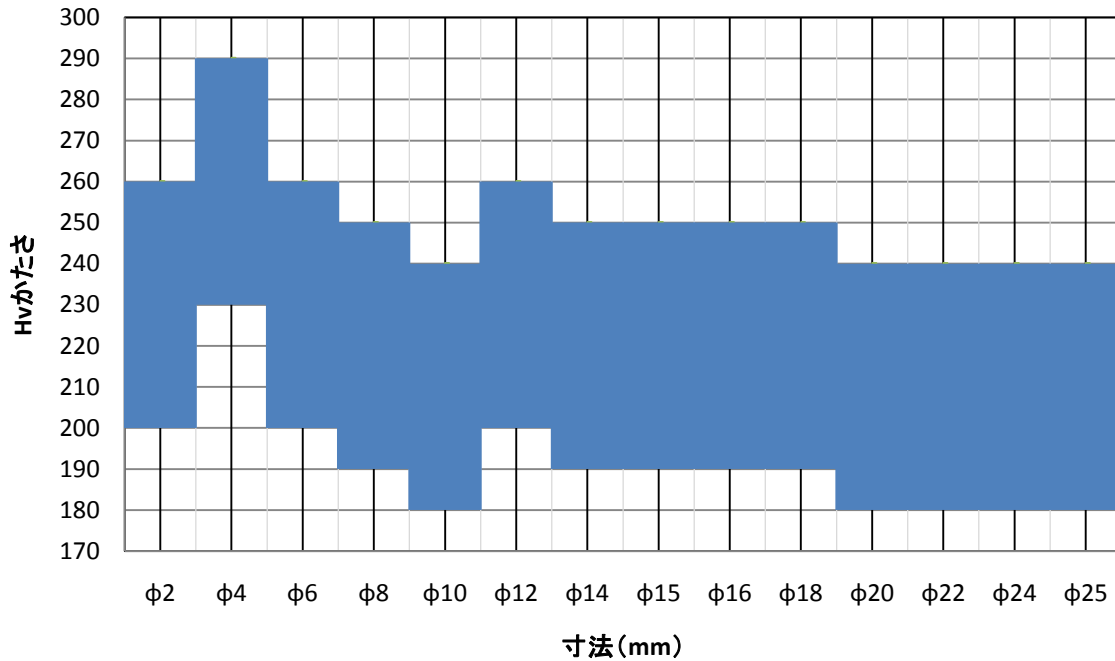
SF27E(SUS303Cu)-D 寸法別機械的性質:Hvかたさ(測定位置:中心)
