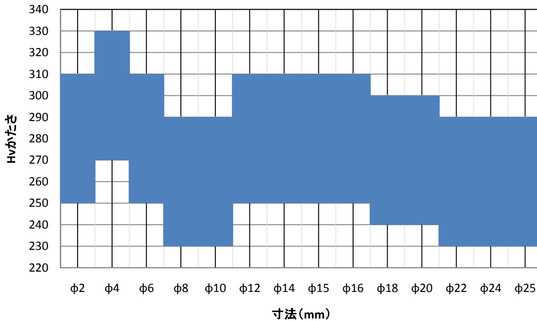
SF27E(SUS303Cu)-D 寸法別機械的性質:Hvかたさ(測定位置:表層部)
