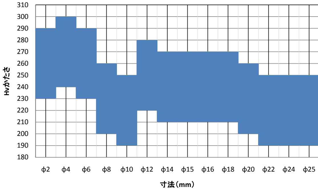
SF27E(SUS303Cu)-D 寸法別機械的性質:Hvかたさ(測定位置:直径/4)
