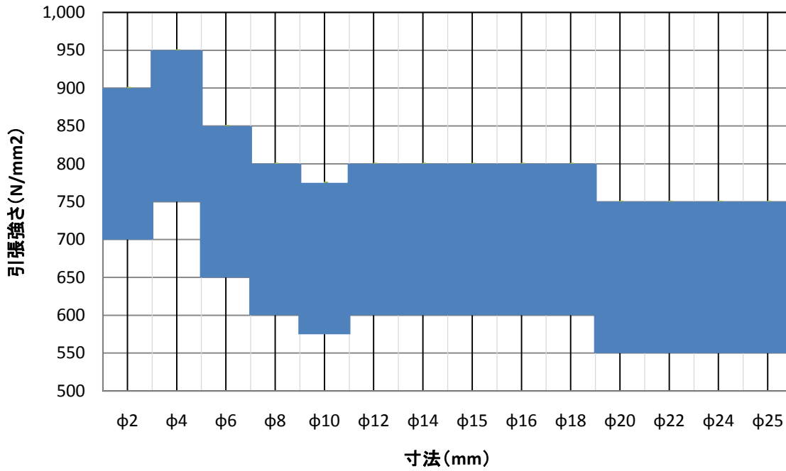
SF27E(SUS303Cu)-D 寸法別機械的性質:引張強さ
