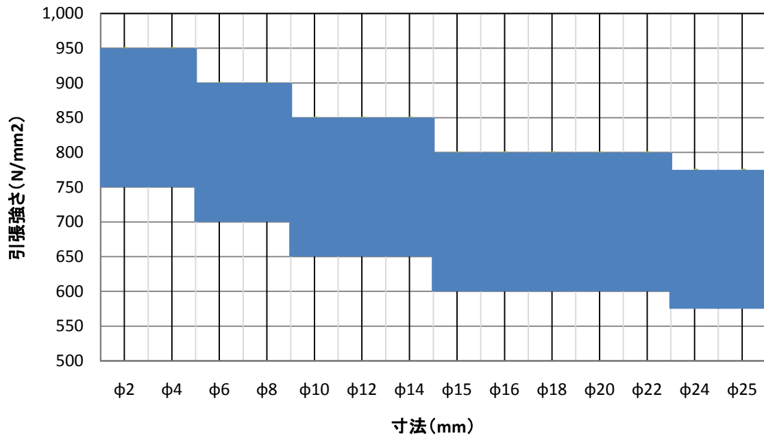
SUS420系-D 寸法別機械的性質:引張強さ (SF53-E, SUS420F, SUS420F2)
