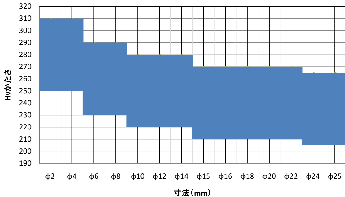
SUS420系-D 寸法別機械的性質:Hvかたさ (SF53-E, SUS420F, SUS420F2)
